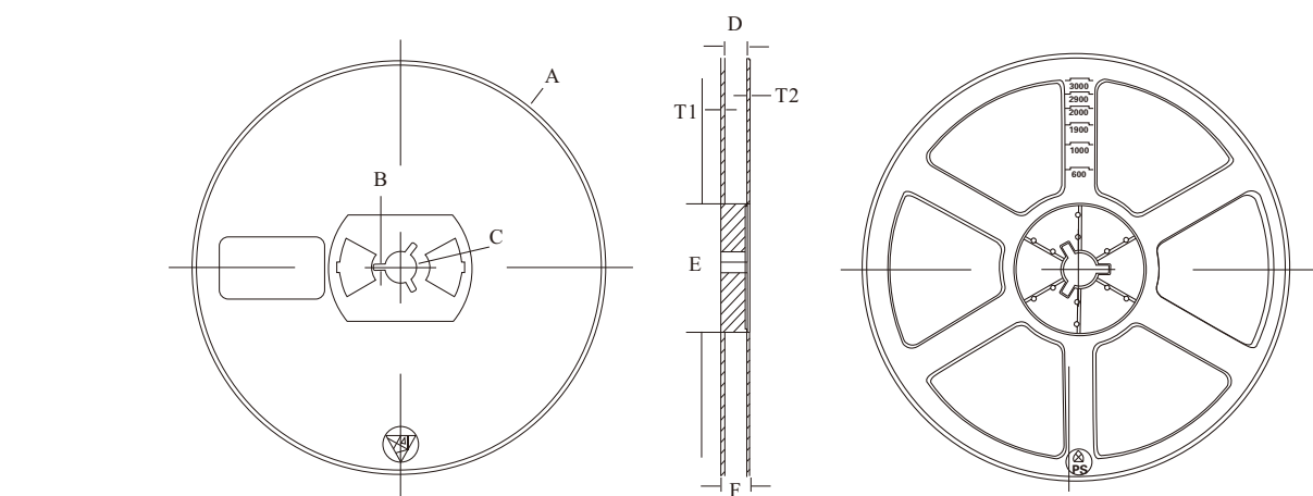
Reel (7")
